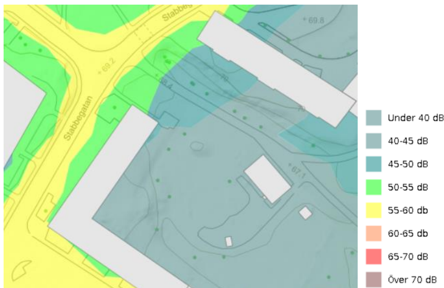
Trafikbuller utbredning ekvivalentnivå, 2018 års trafikdata
